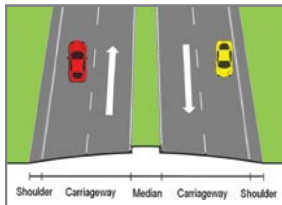
चित्र 1.4 सड़क का आदर्श अनुप्रस्थ काट (क्रॉस-सेक्शन)
