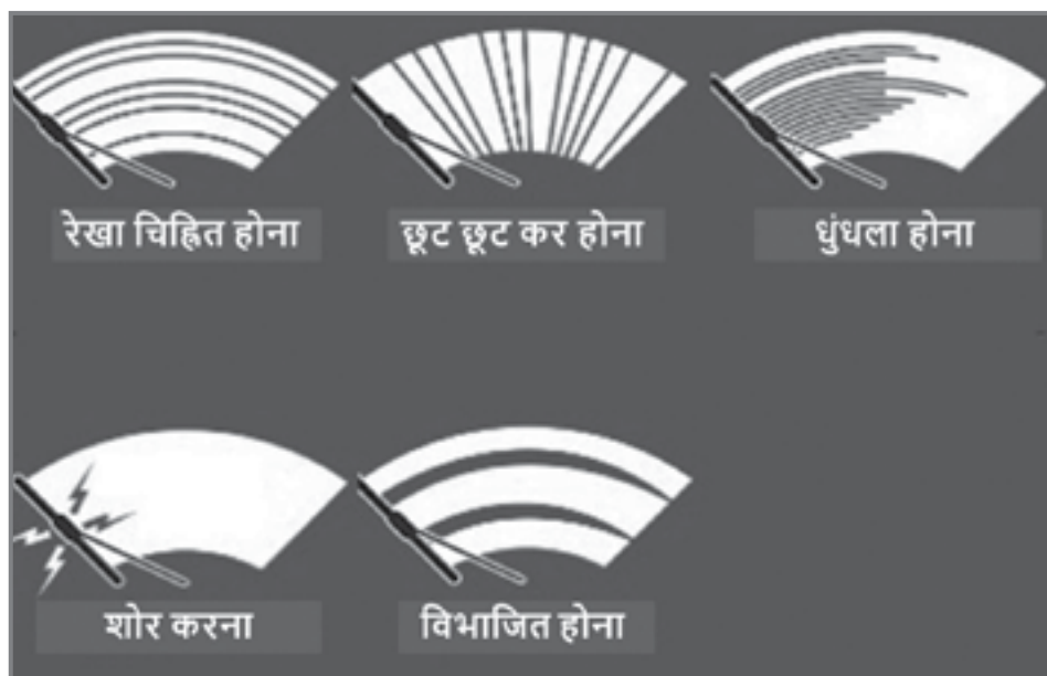
चित्र 5.9: वाइपर ब्लेड की आम समस्याएँ
