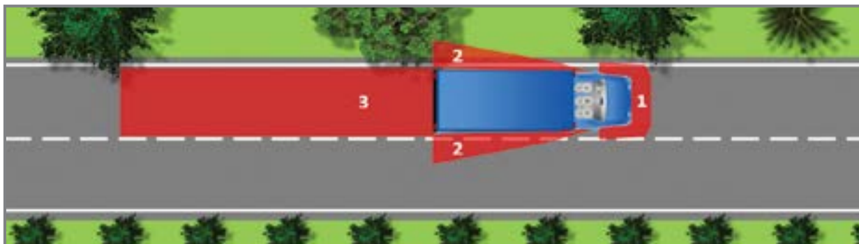
चित्र 4.42: भारी वाहन के ब्लाइंड स्पॉट
